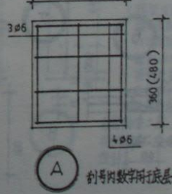
水冲槽式厕所便槽详图
