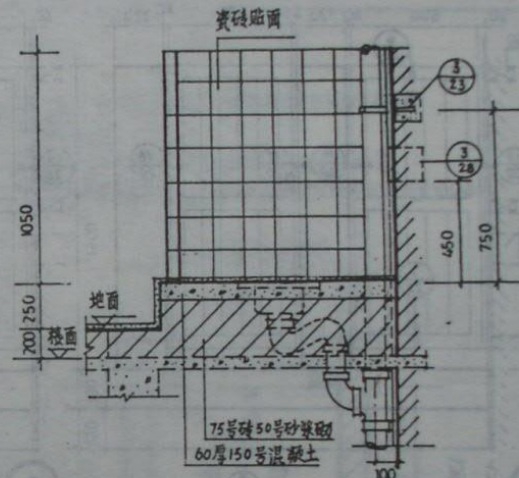
1-1剖面
