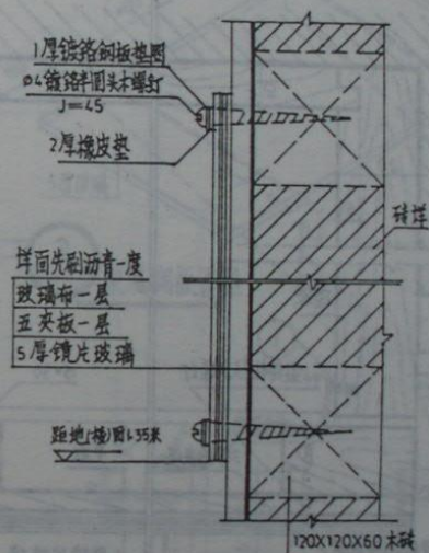
1-1 剖面
