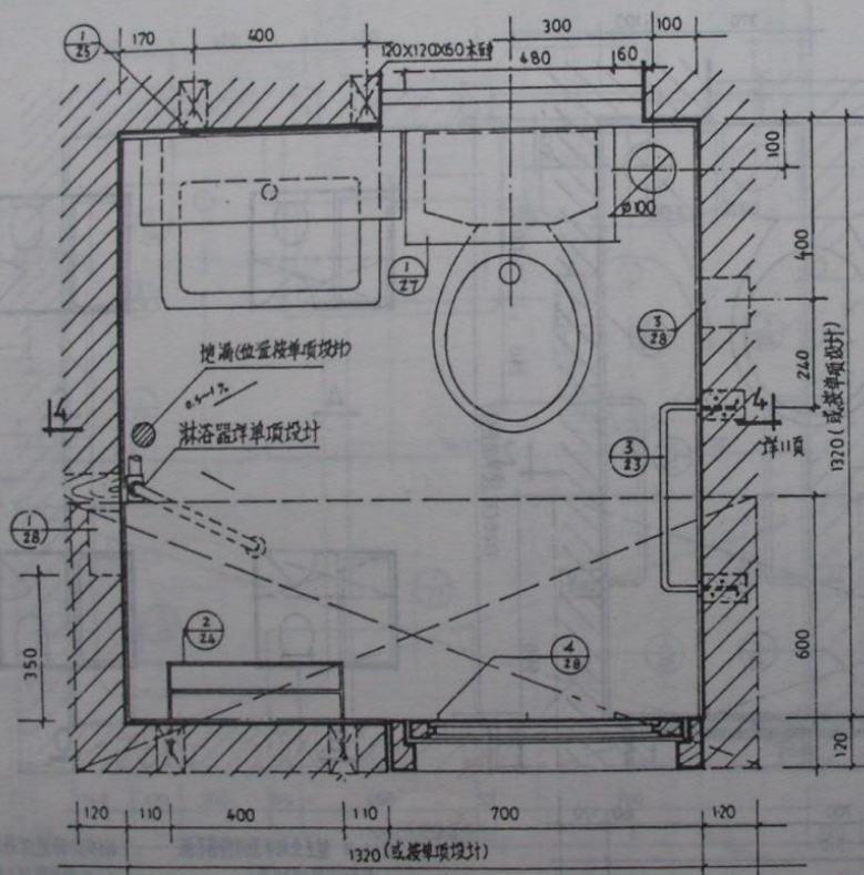
卫生间平面
