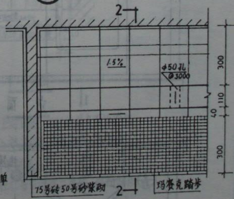
② 平面
