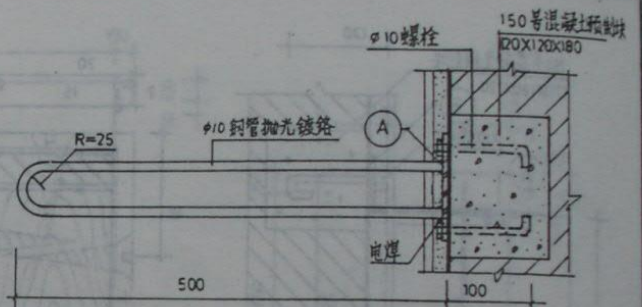
1 镀铬钢管毛巾架
