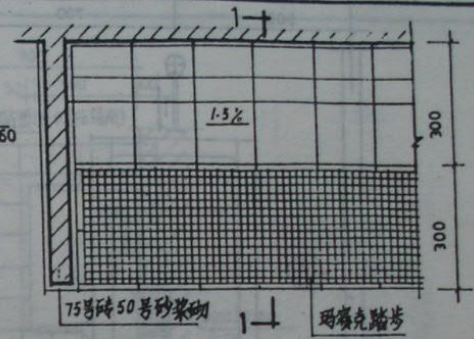
① 平面
