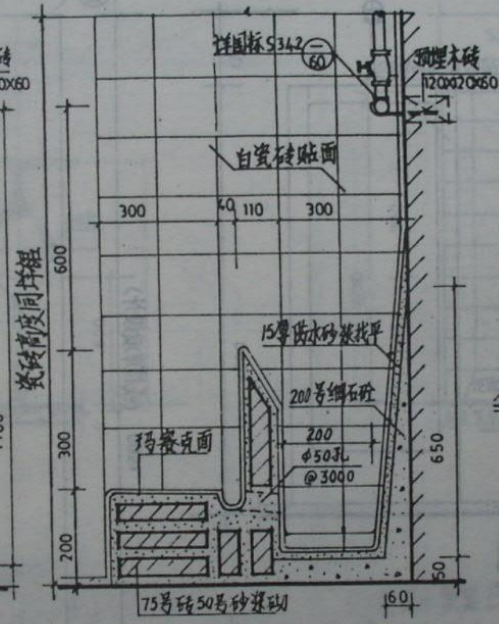
2-2剖面
