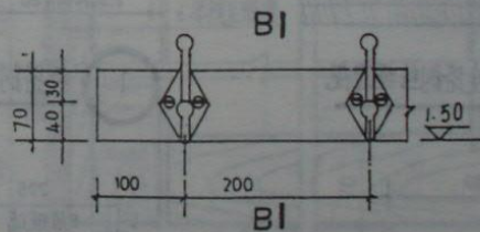
4 成品挂衣钩
