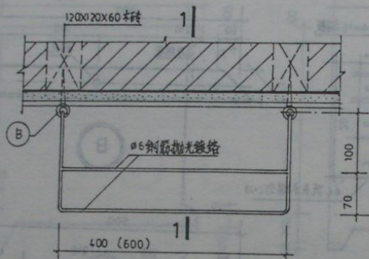
2 6mm 钢筋镀铬毛巾架
