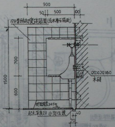
1-1 剖面
