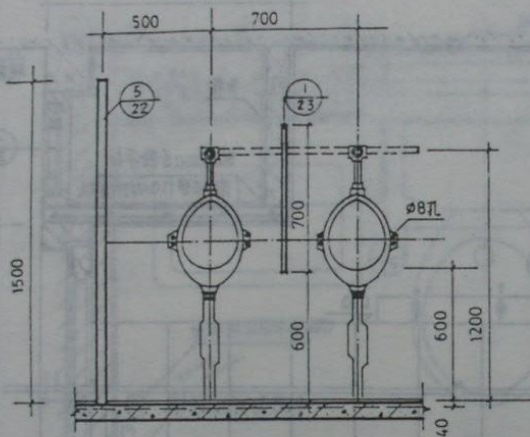
立面
