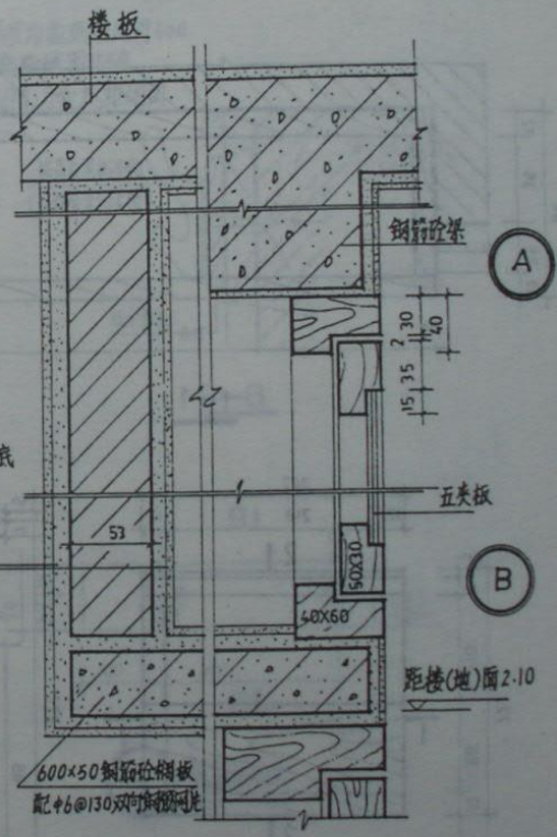
卫生间吊柜详图
