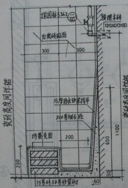
1-1剖面
