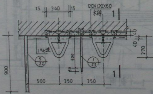
平面
