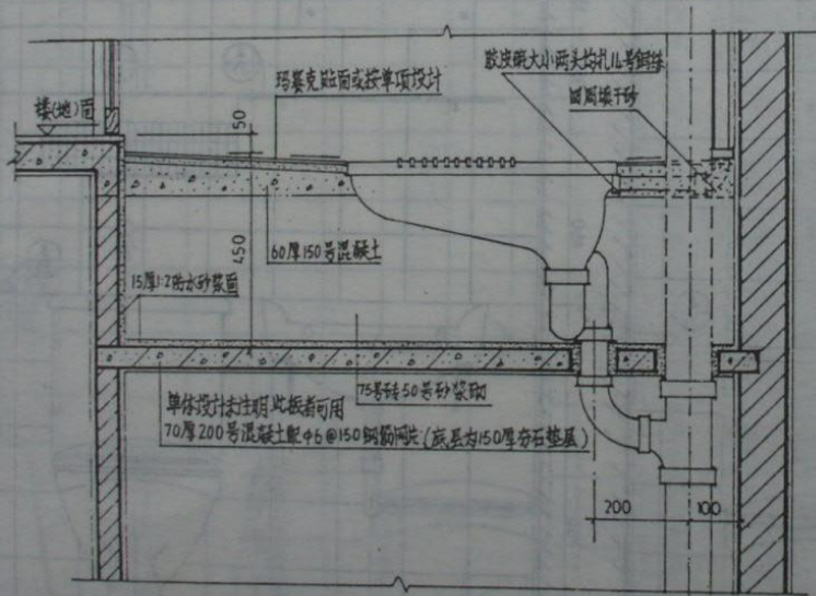
1-1剖面
