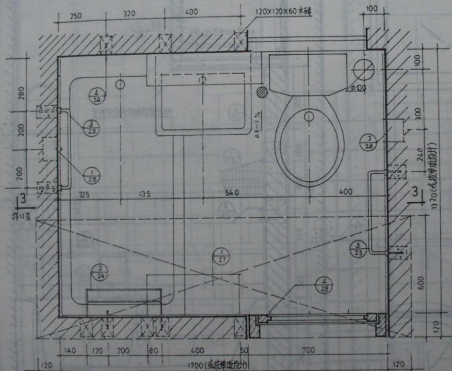
卫生间平面
